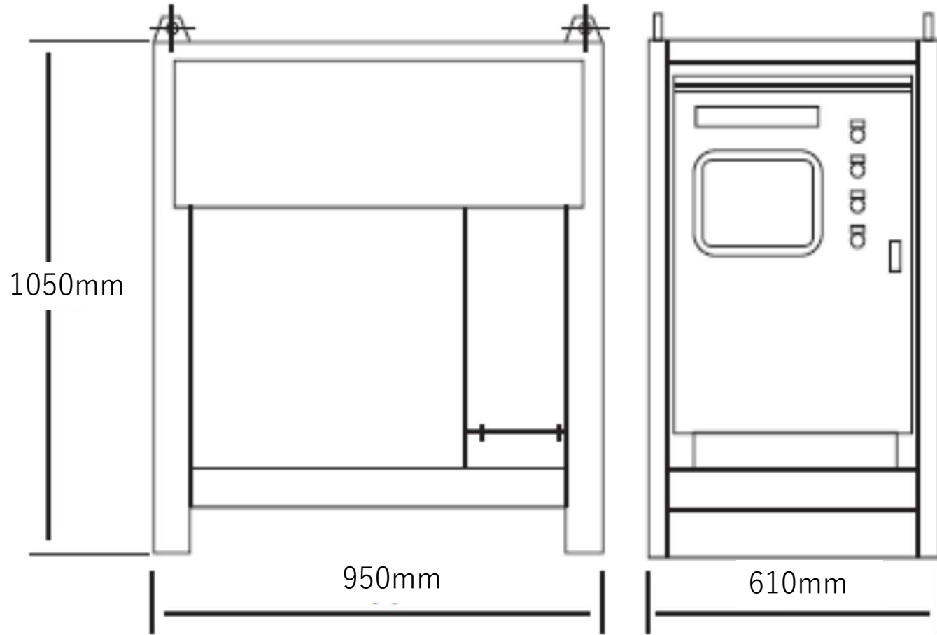
型式NTN-6NB 外形図
