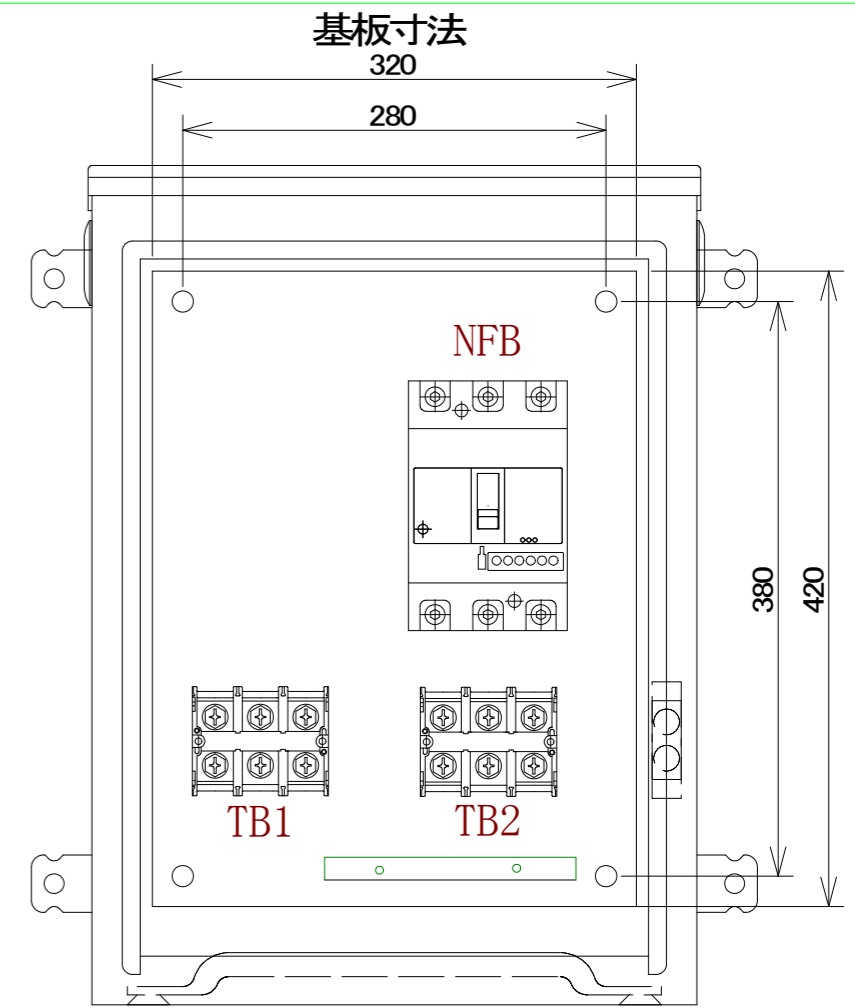
配置図
