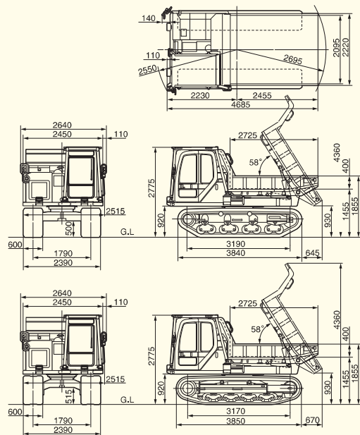
■一体型ゴムシュー仕様車 CD60R-1A
