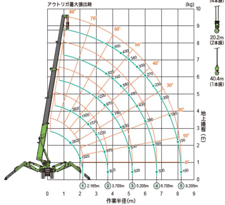
作業半径・揚程図 (4本掛け時)
