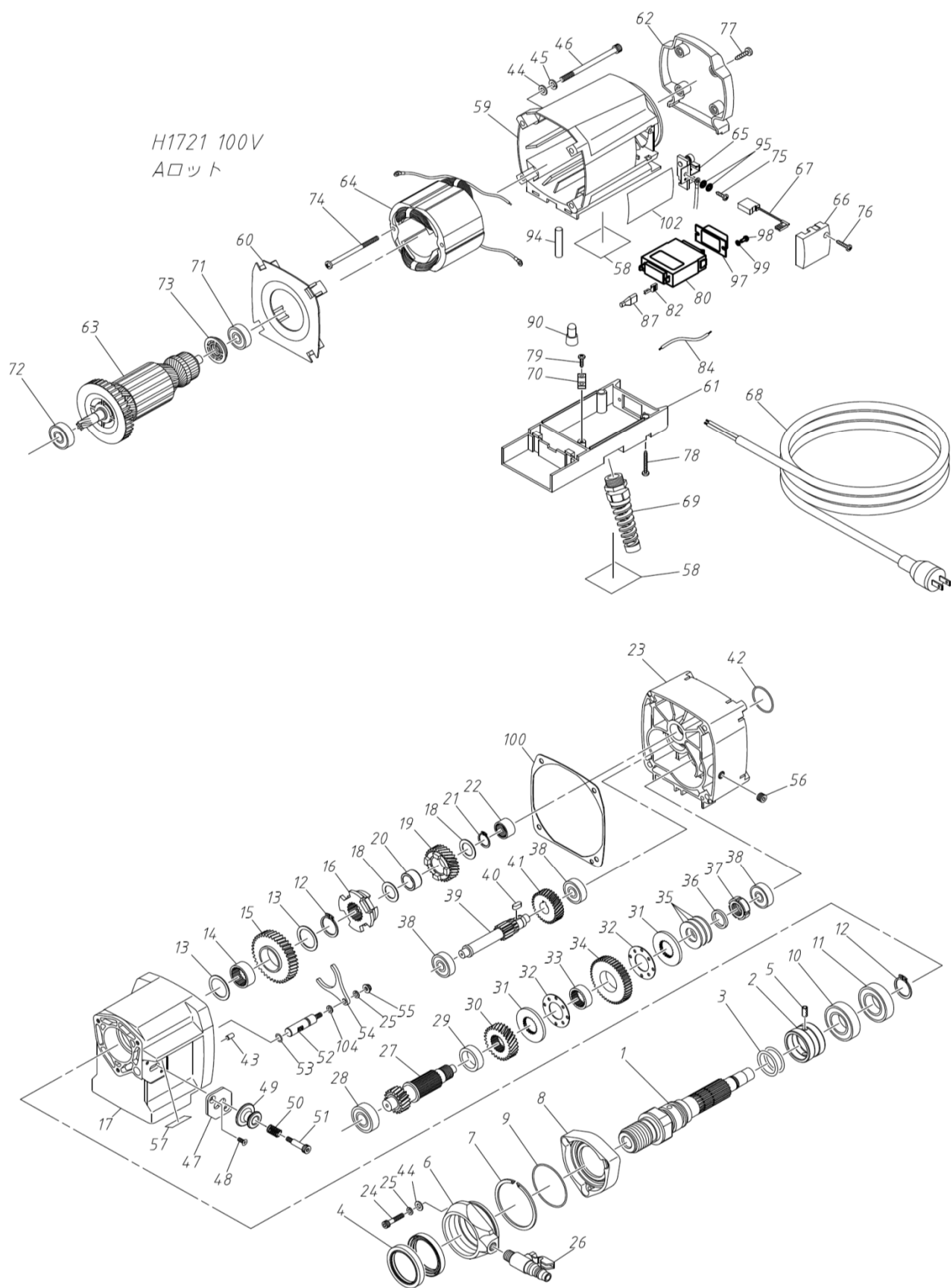
H1721 100V A口ッ 部品構成図
