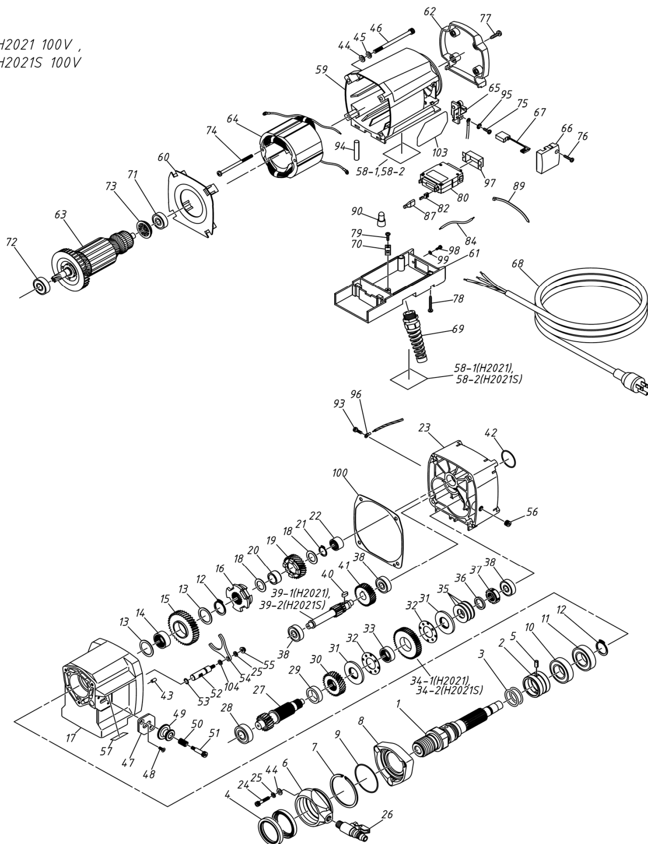
H2021(TS-255PRO),H2021S(TS-255PRO SPEED) 部品構成図
