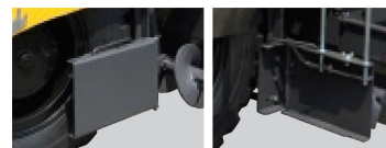
折畳式リネーティングプレート(閉状態) 折畳式リネーティングプレート(開状態)
