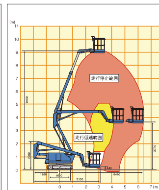
■NUL090-6作業範囲図
