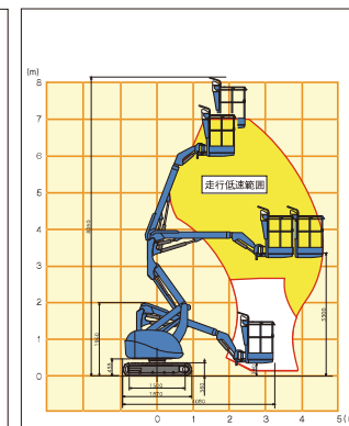
■NUL070R-2作業範囲図
