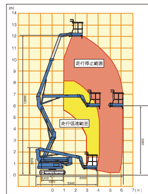
■NUL120-6作業範囲図
