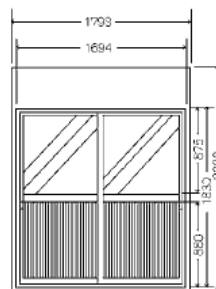
⑨両引戸パネル (HD)
