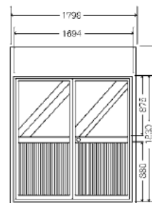
⑩両開きドアパネル (RD)
