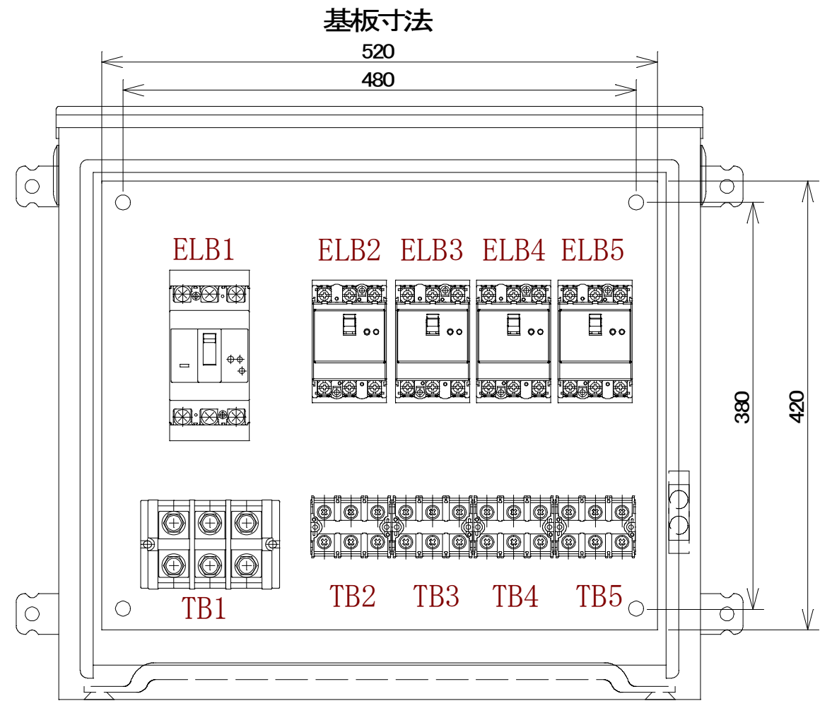
配置図
