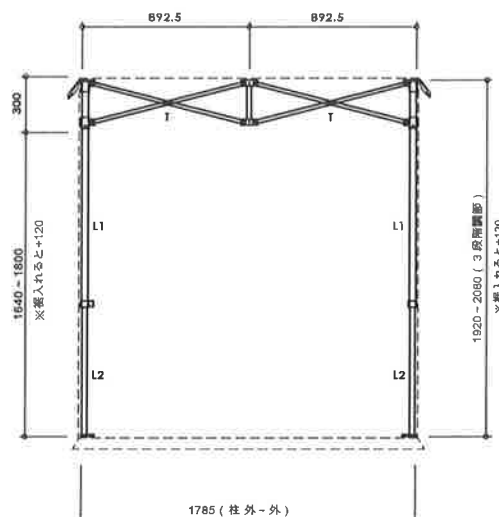
軸組図 (3正面)
