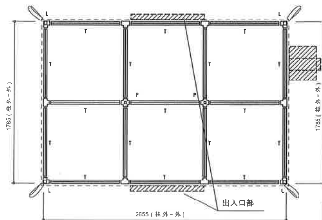
伏図
