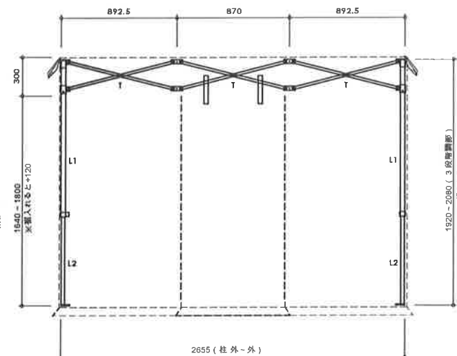
軸組図 (4正面向かって右)
