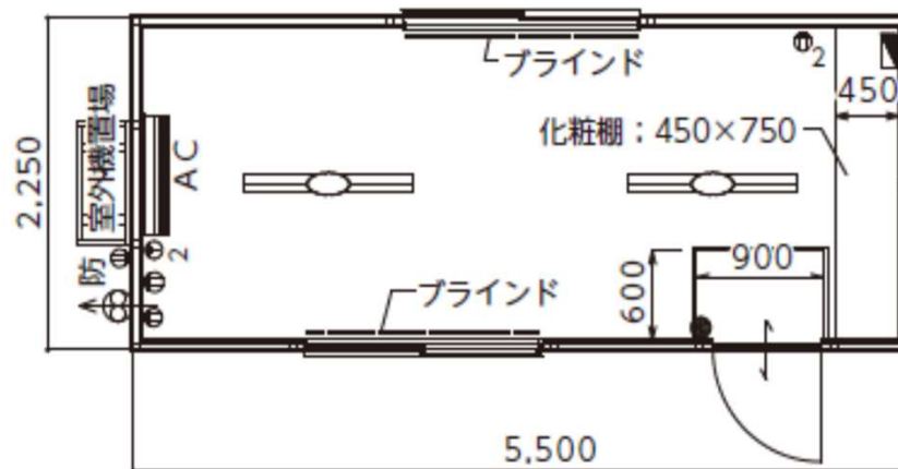
■平面図(床置き設置型4坪エアコン付)
