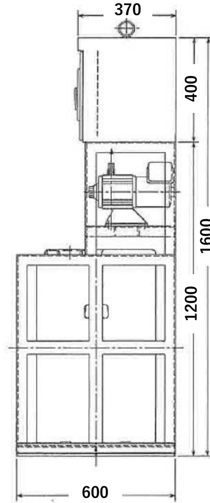
右側面図
