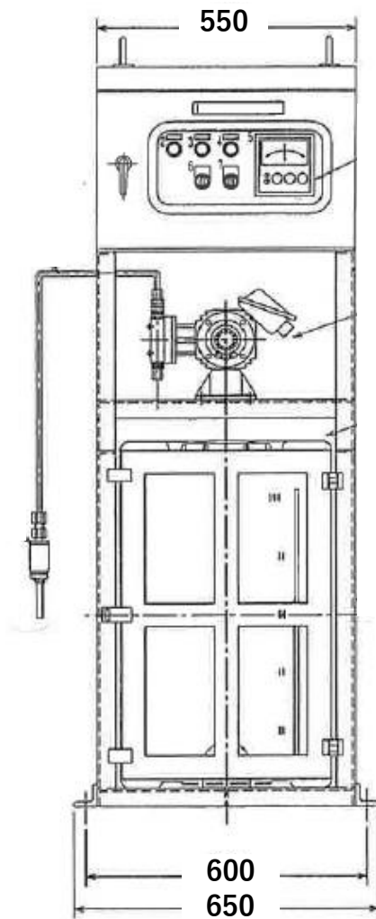
正面図
