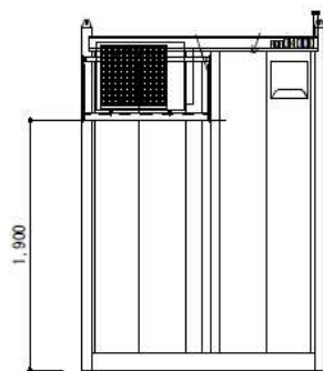
X1立面図 S=1/50
