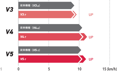
登坂速度比較
