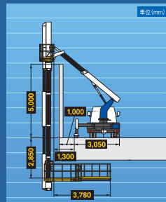
アウトリガ: 最大張出
