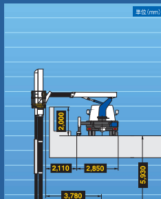
アウトリガ: 中間2張出
