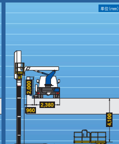
アウトリガ: 中間1張出
