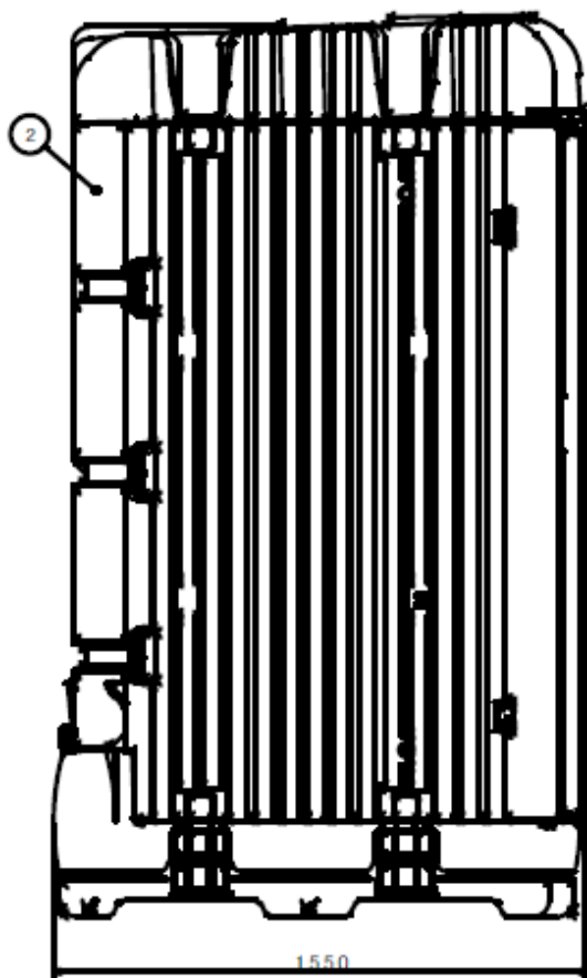
左側面図
