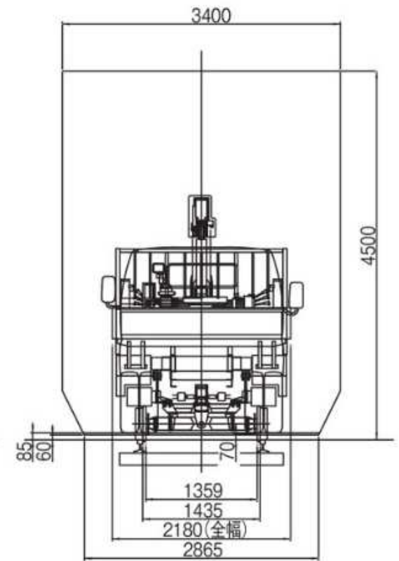
【車両限界寸法/新幹線】
