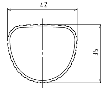
踏ザン断面図
