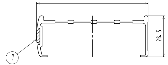
支柱断面図
