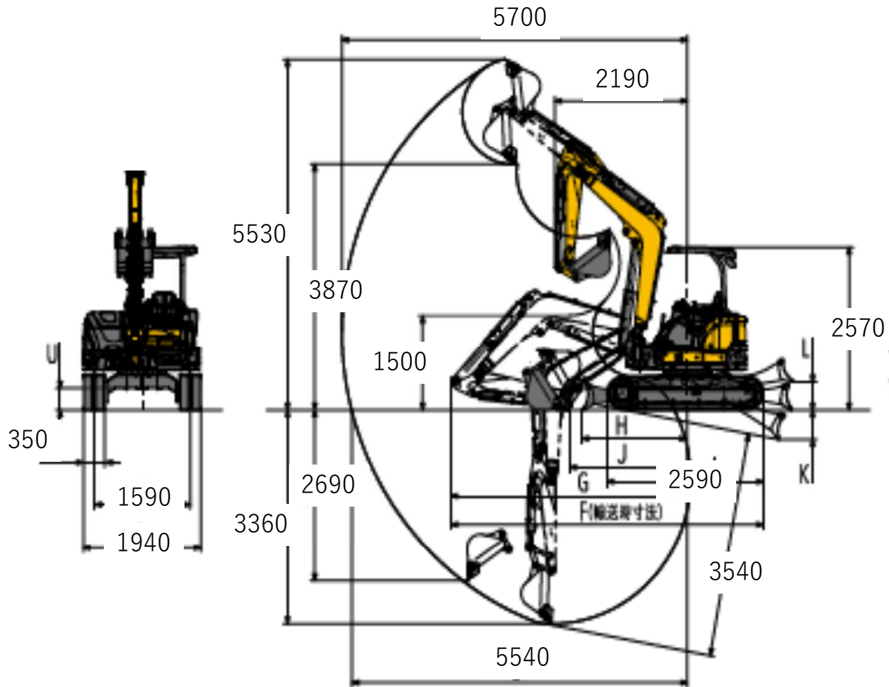
VIO45-6A外形图 (单位：mm)
