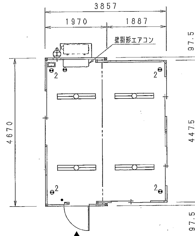
平面図
