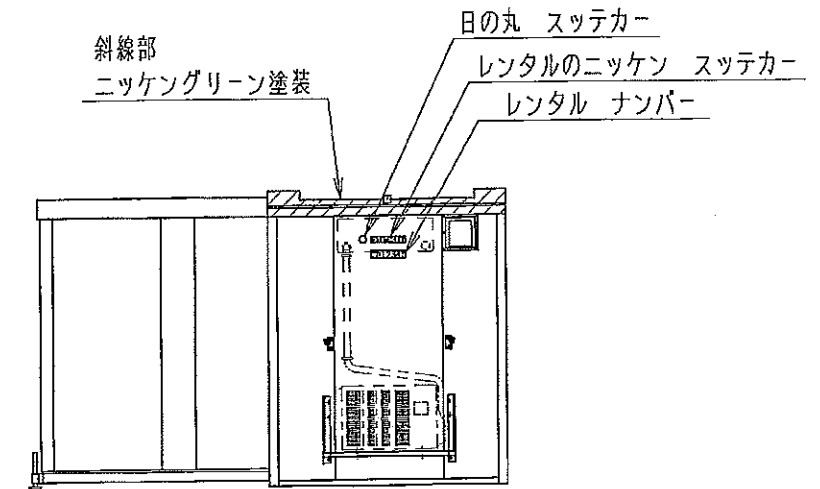
C 立面図
