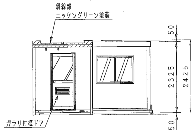
A 立面図
