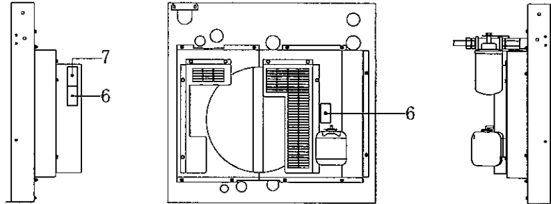
シュラウド部貼付け位置
