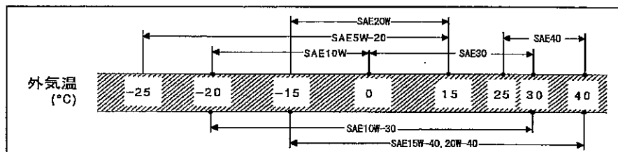
使用外気温の範囲と粘度 (SAE)
