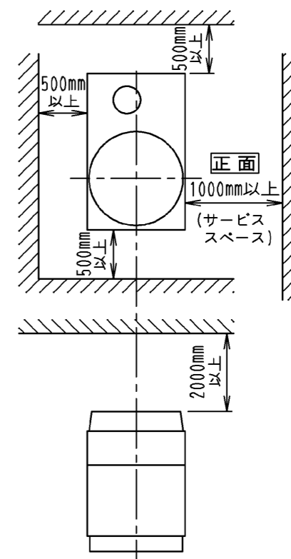
〈据付サービススペース〉
