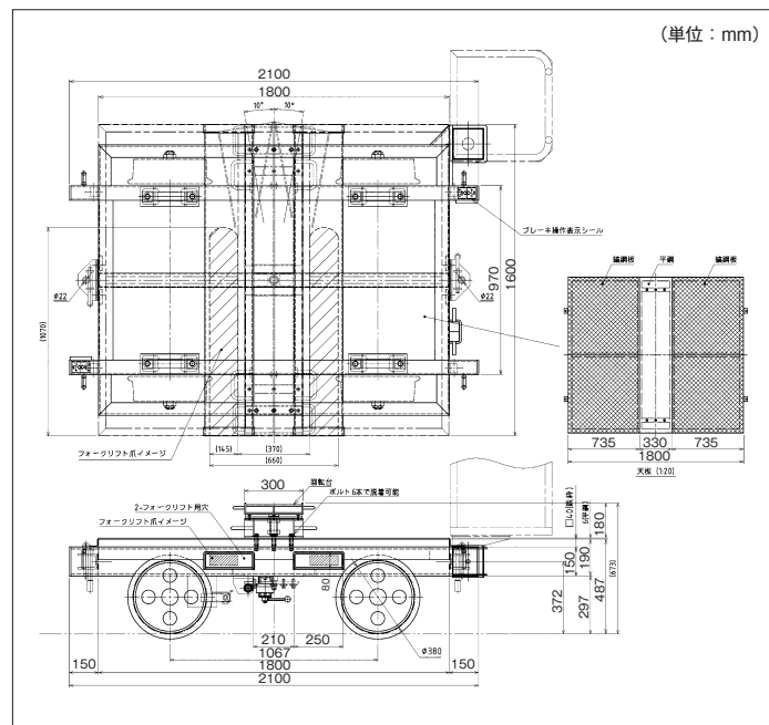
■外形図：保線機器整備製 2.7t 狭軌
