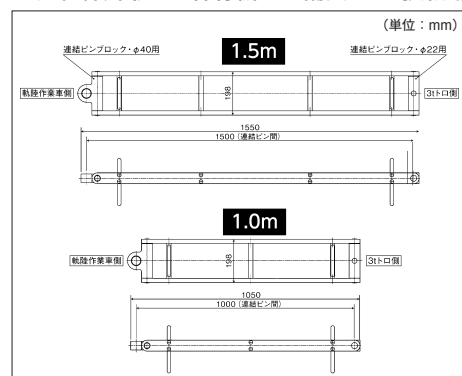
■連結棒外形図：保線機器整備製 2.7t 狭軌用
