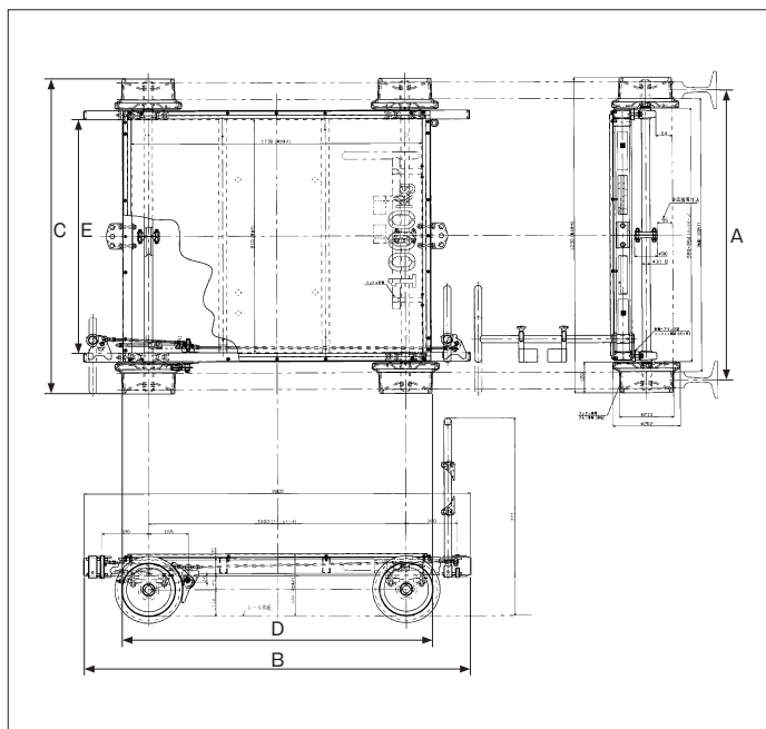
■仕様 (0.5 ~ 1t)
