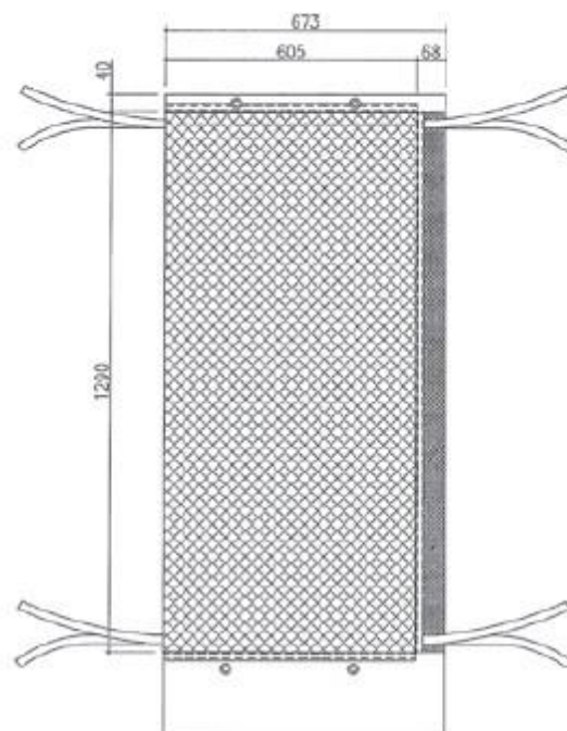
パネル形状図(音源側)
