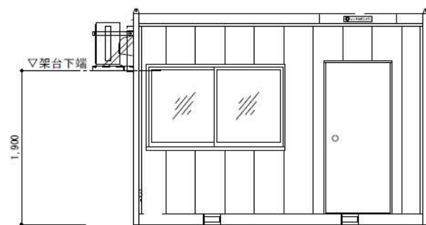
Y 1 立面図 S=1/50
