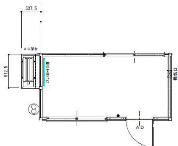
平面図 S=1/50
