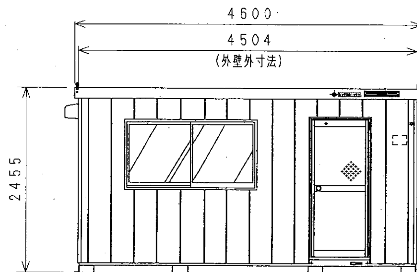
A立面図 S=1/50
