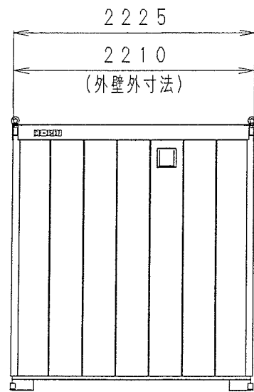
B 立面図
