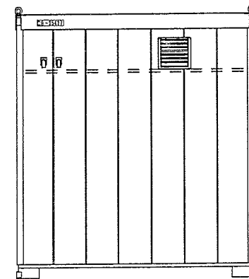
D 立面図
