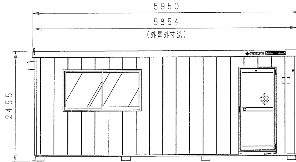
A 立面図
