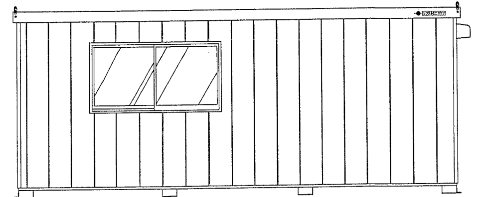
C 立面図
