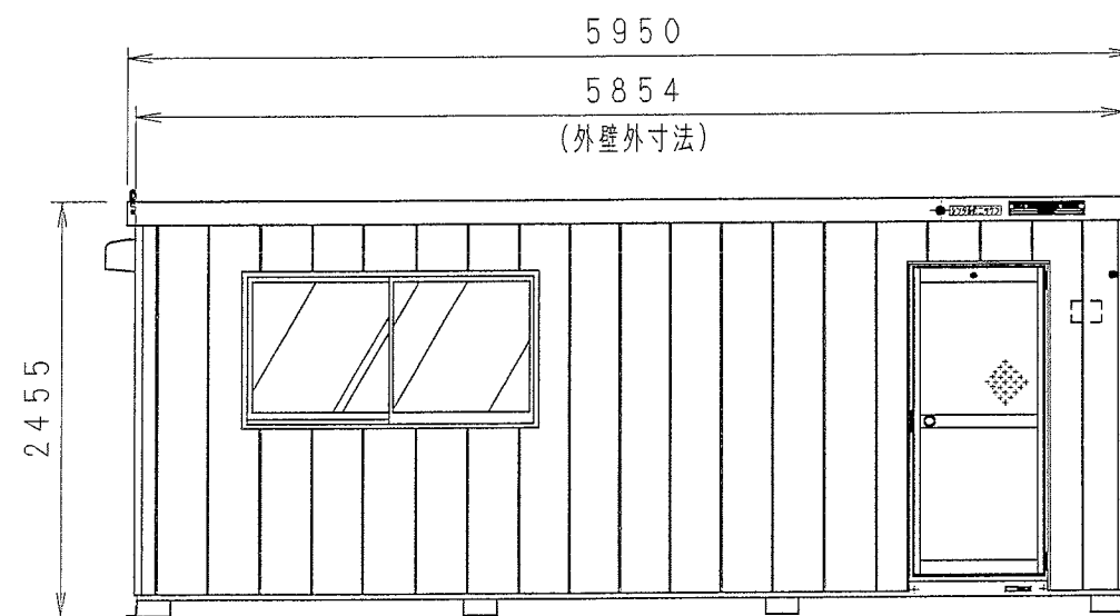
A 立面図 S=1/50
