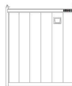
X2 立面図 S=1/50
