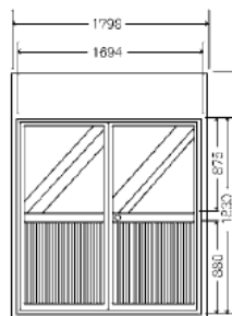
⑩両開きドアパネル (RD)
