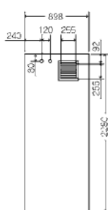
②換気パネル (K)
