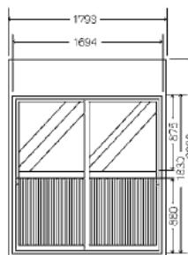
⑨両引戸パネル (HD)
