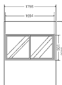
⑥窓Lパネル (L)
