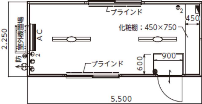
■平面図(床置き設置型4坪エアコン付)
