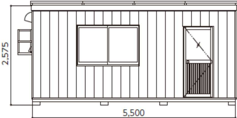
■立面図(床置き設置型4坪エアコン付) (単位: mm)
