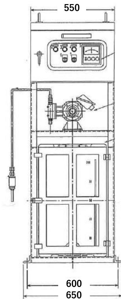
正面図
