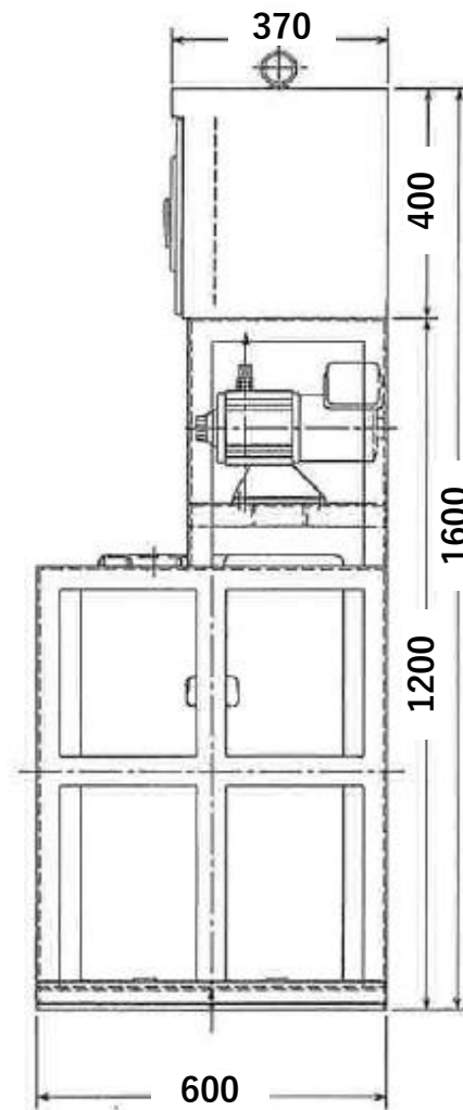
右側面図
