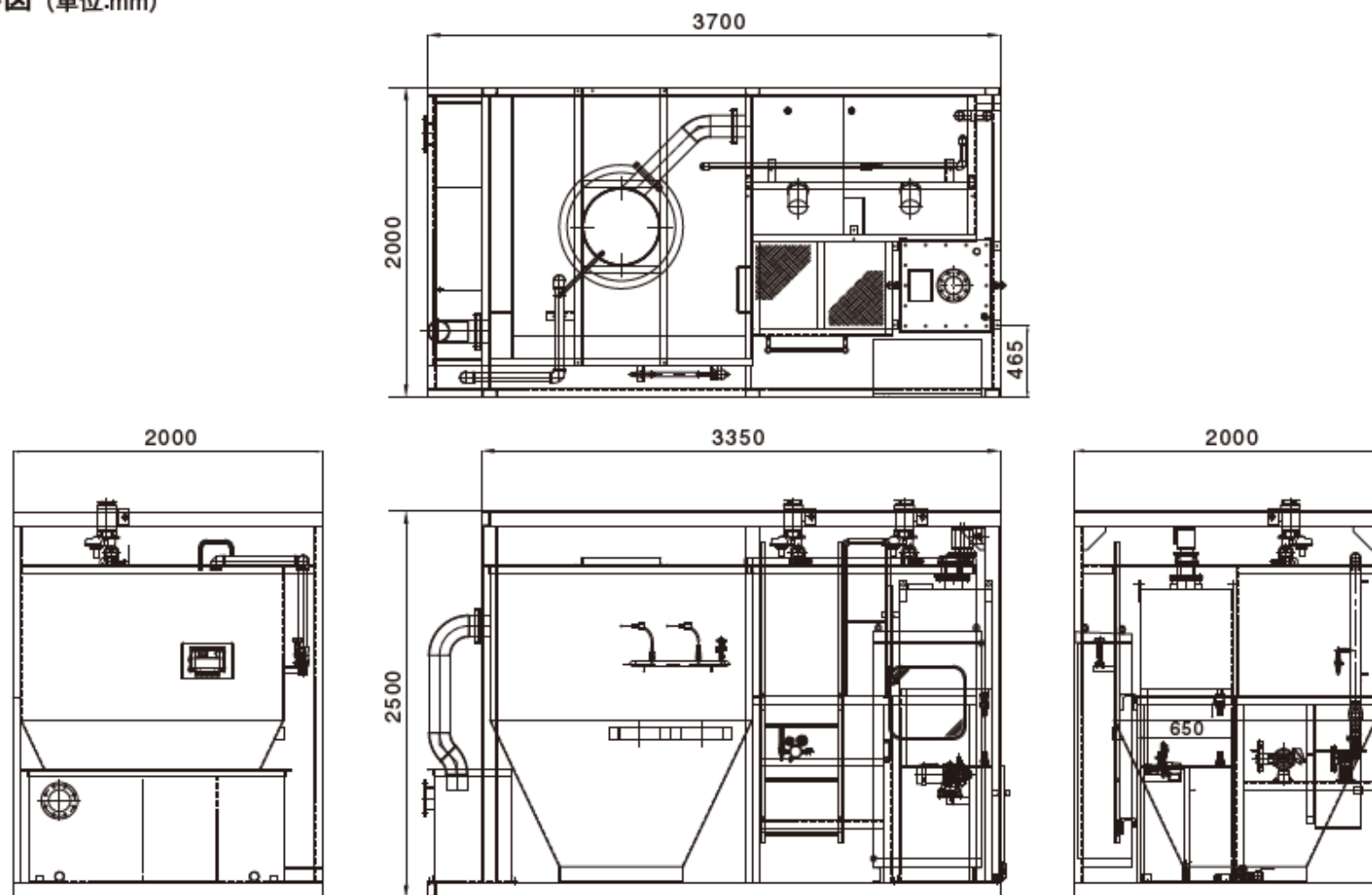
外形図 (単位:mm)
