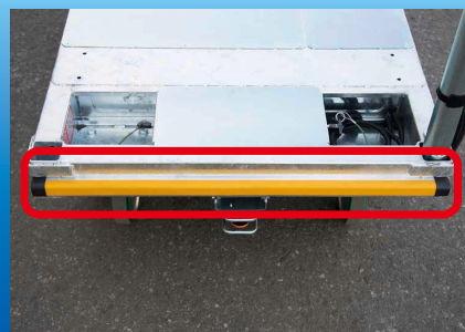
衝突停止バンパースイッチ (前後)
