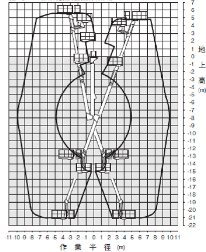
第3ブーム作業範囲(壁面作業図)
