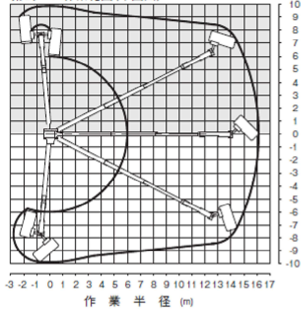
第3ブーム作業範囲(平面図)
