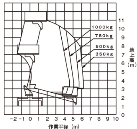
アウトリガ張出幅 中間2（ジャッキベース使用時）
