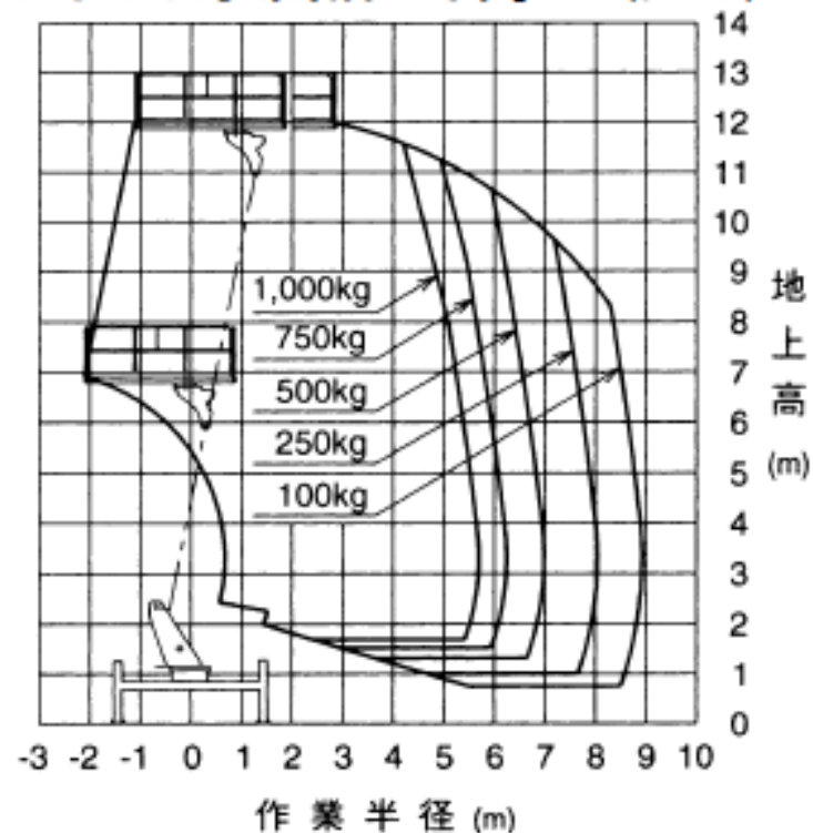
アウトリガ張出幅 中間 2 (側方)
