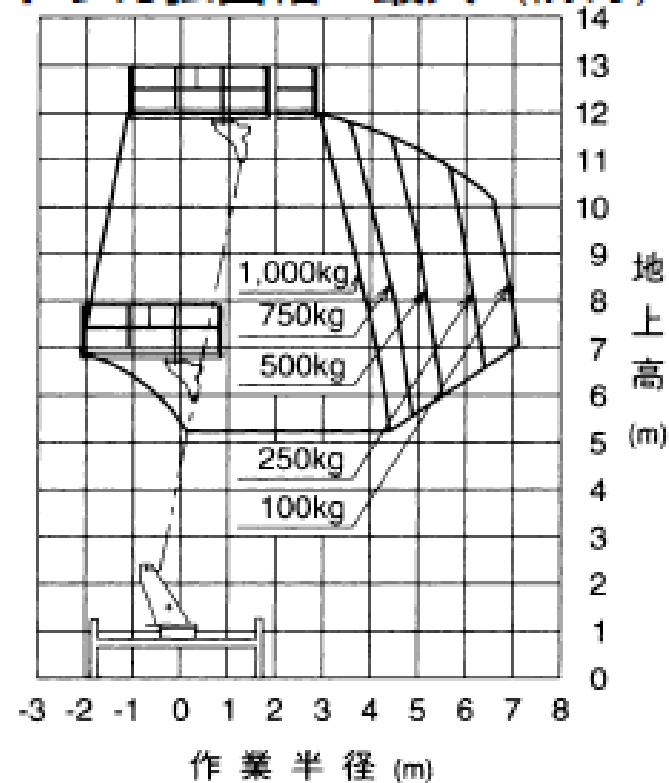
アウトリガ張出幅 最大 (前方)
