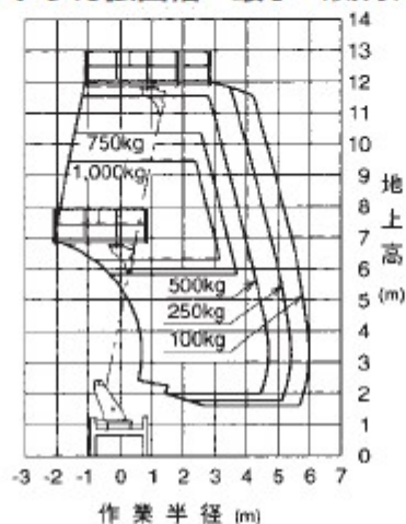
アウトリガ張出幅 中間 1 (側方)
