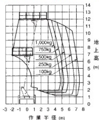
アウトリガ張出幅 中間 1 (側方)
