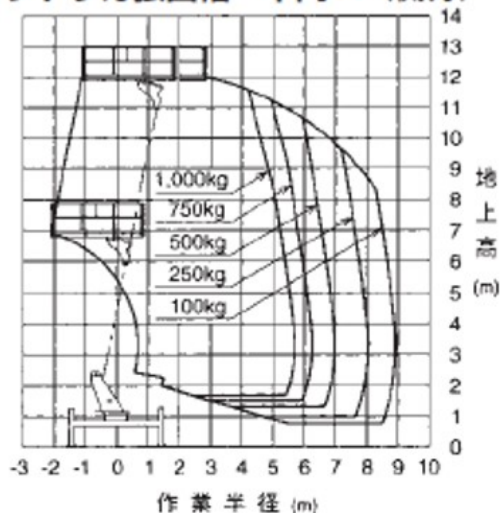
アウトリガ張出幅 最大 (前方)
