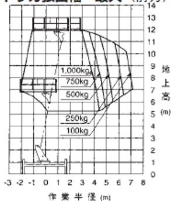
アウトリガ張出幅 最大 (前方)
