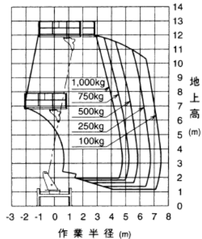
アウトリガ張出幅 中間 1 (側方)
