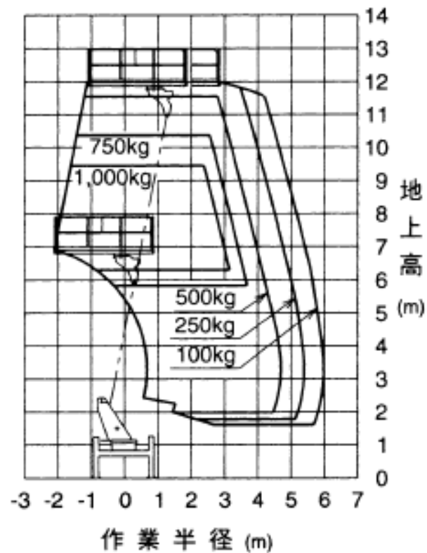
アウトリガ張出幅 最小 (側方)
