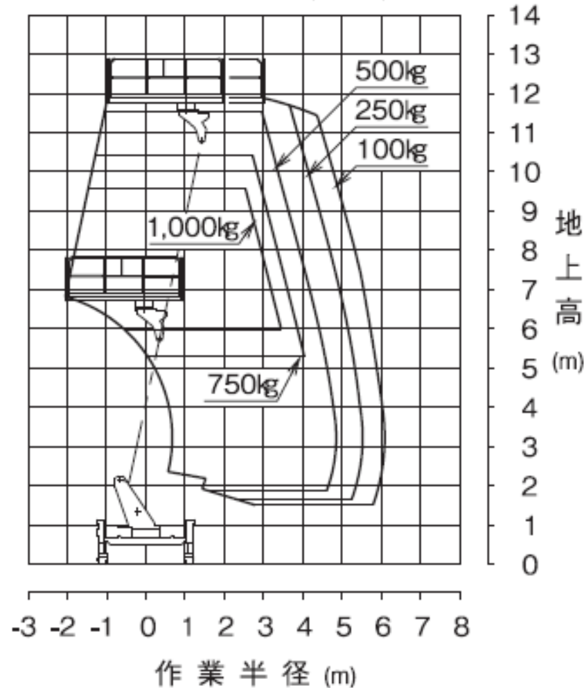
アウトリガ中間1張出(側方)
