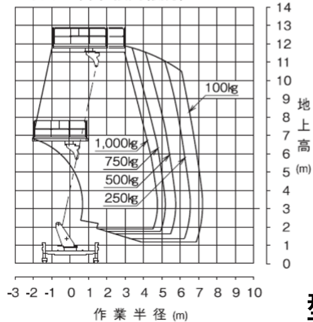
アウトリガ中間2張出(側方)
