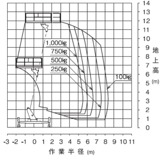
アウトリガ中間2張出(側方)
