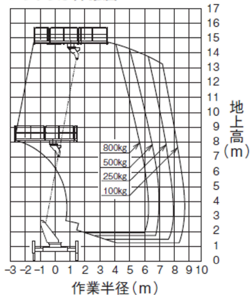
アウトリガ中間張出
