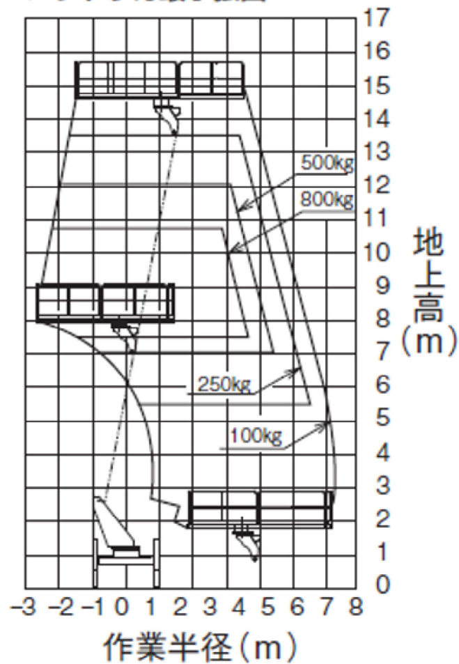
アウトリガ最小張出
