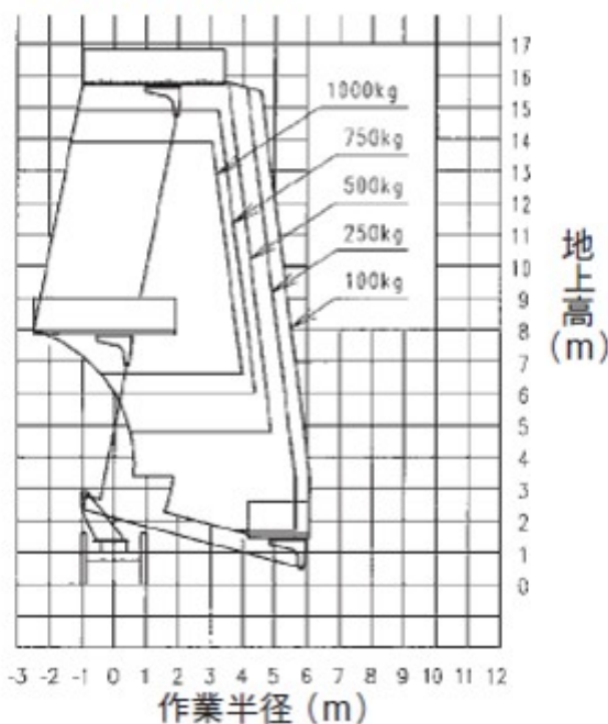
アウトリガ中間1張出
