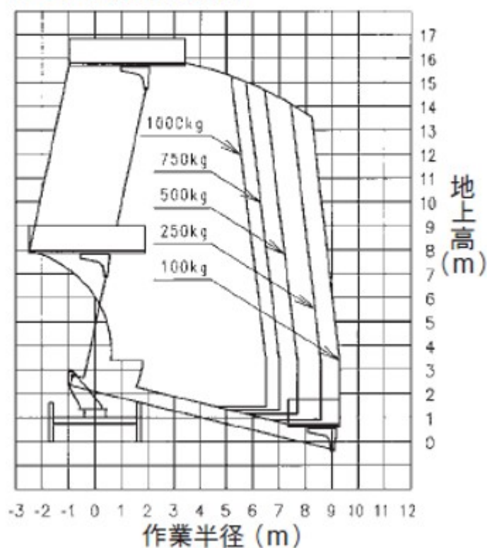
アウトリガ最大張出
