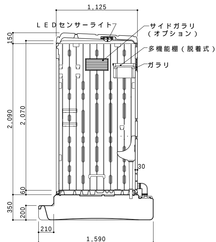
断面図 S=1/30
