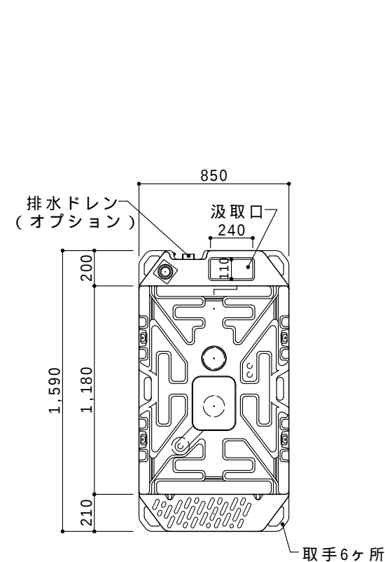
平面図 S=1/30
