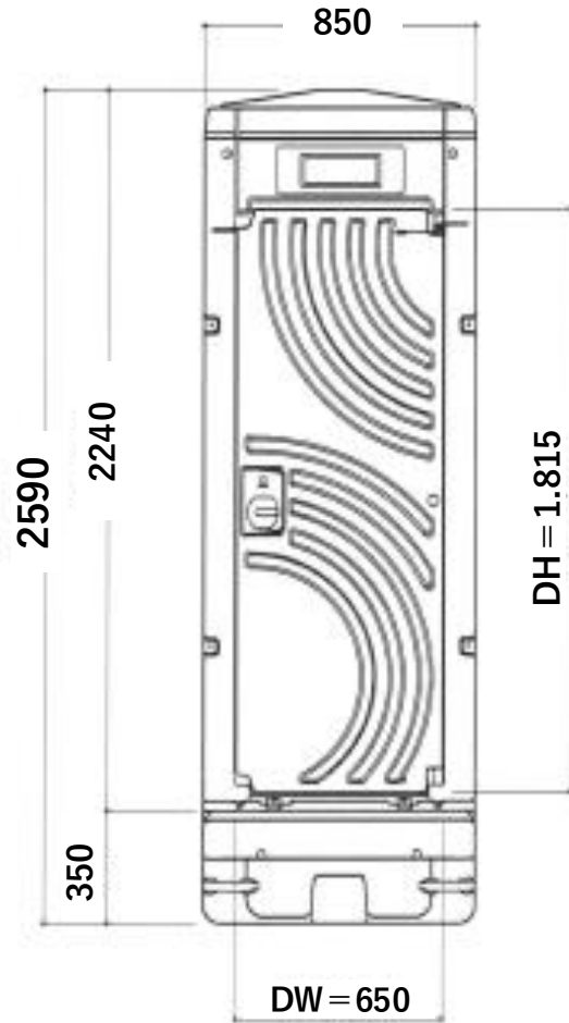
A 立面图 S=1/30
