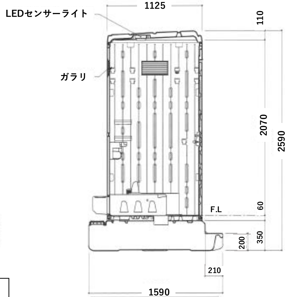
断面図 S = 1/30
