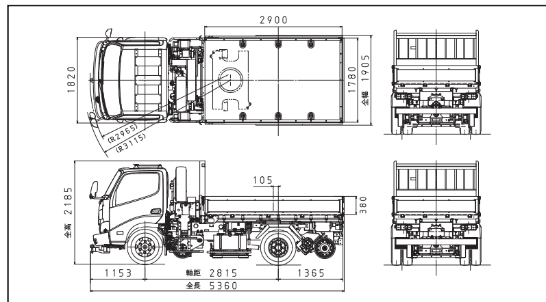
■外形図 (単位:mm)
